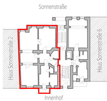
Übersicht EG
